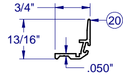
INTERLOCK S-2001
