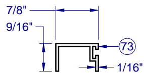
REINF., IMPACT HOOK - 1112
