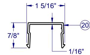
PVC SASH STOP - 6025
