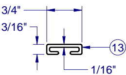
REINF. S.B.R./S.S.R. - 1498
