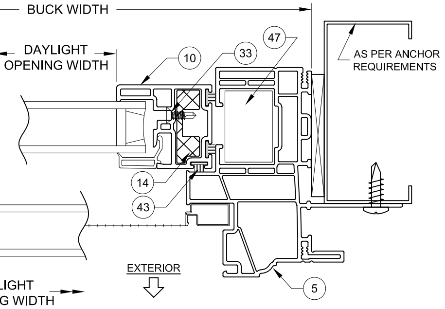
5 FIN FRAME X-SECTION STEEL STUD CONSTRUCTION
