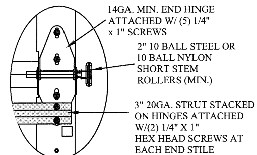
TYPICAL END HINGE N.T.S. 3
