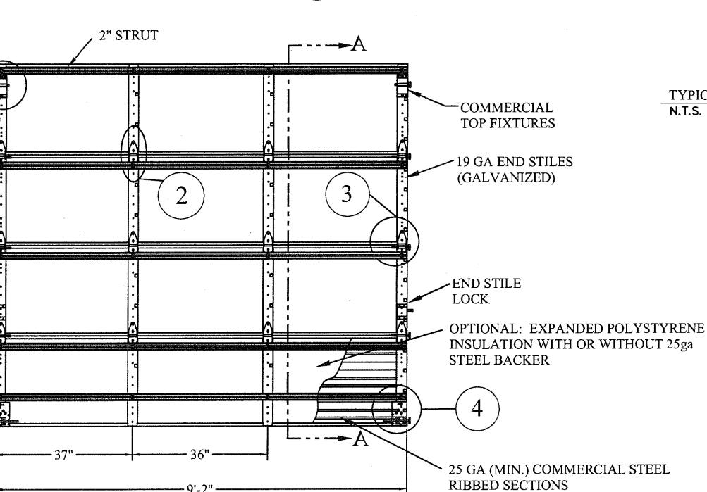
DOOR INTERIOR ELEVATION N.T.S.
