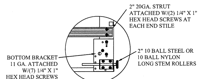
TYPICAL BOTTOM BRACKET N.T.S. 4
