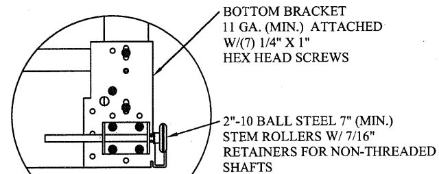
TYPICAL BOTTOM BRACKET N.T.S.
