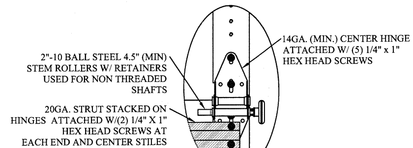
TYPICAL END HINGE N.T.S.
