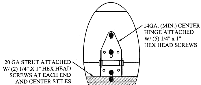
TYPICAL CENTER HINGE N.T.S.
