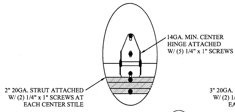
EVEN SECTION CENTER HINGE N.T.S. 2
