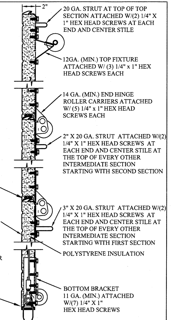
SECTION A-A (SIDE VIEW) N.T.S.
