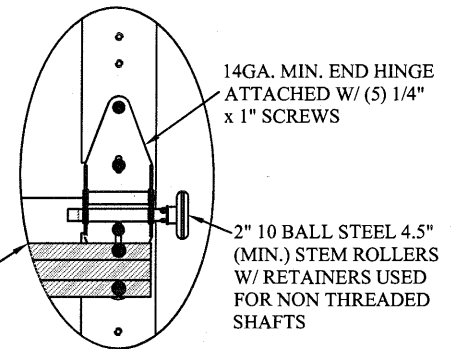
ODD SECTION END HINGE N.T.S. 5
