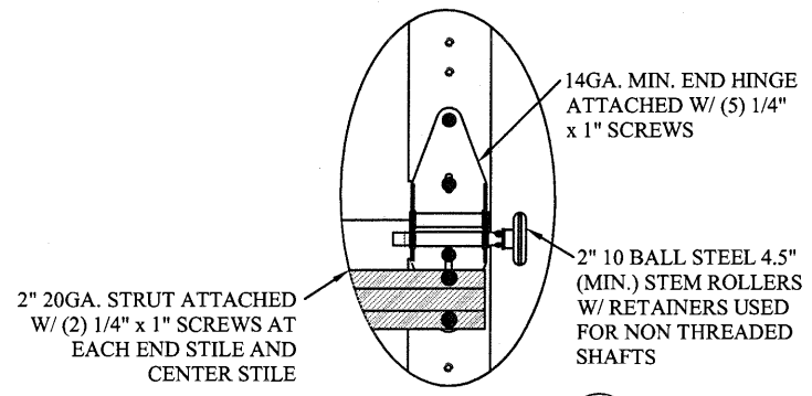
EVEN SECTION END HINGE N.T.S. 4
