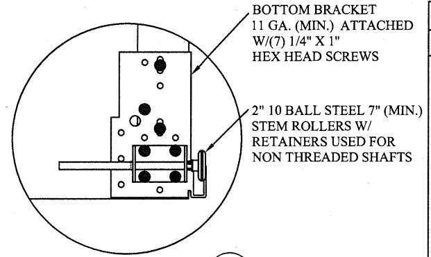
TYPICAL BOTTOM BRACKET N.T.S. 6
