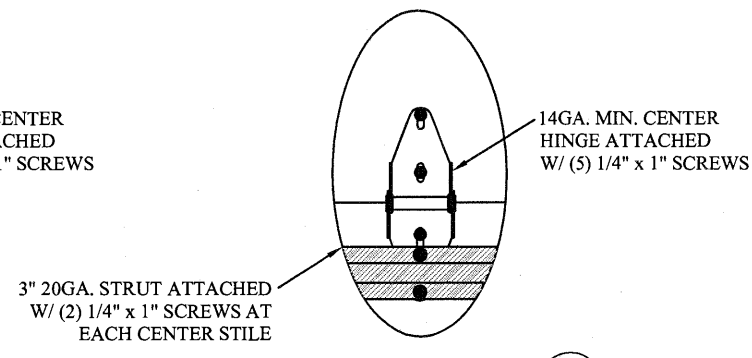
ODD SECTION CENTER HINGE N.T.S. 3
