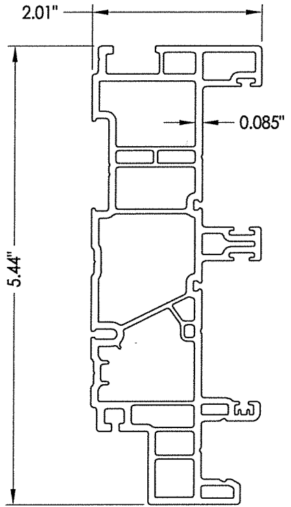
3 FRAME JAMB
