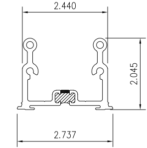
6 FRAME LUG
