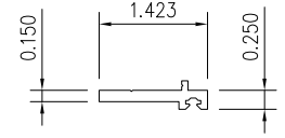
5 FRAME CAP
