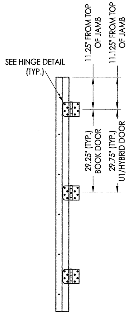
HINGE JAMB
