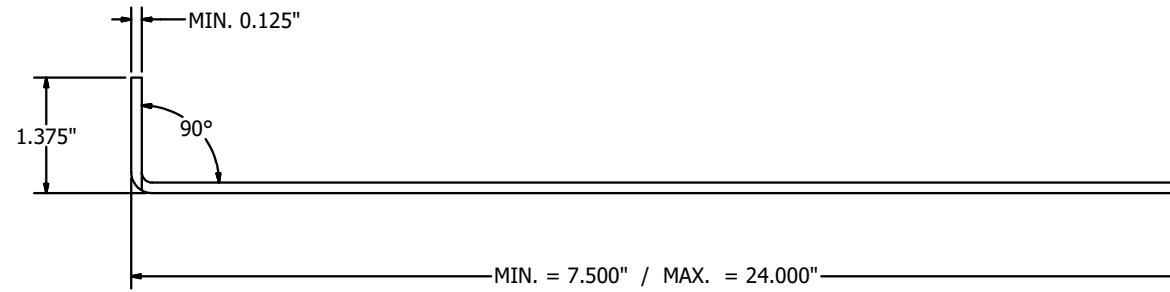
UNIVERSAL SLEEVE ITEM-18 N.T.S.
