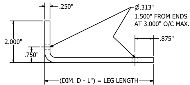
RETAINING ANGLE ITEM-21 N.T.S.
