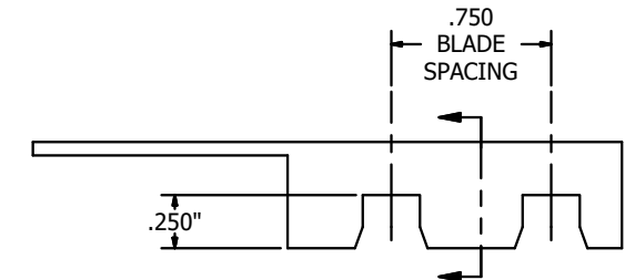
H.H.B.S. ITEM-5 N.T.S.
