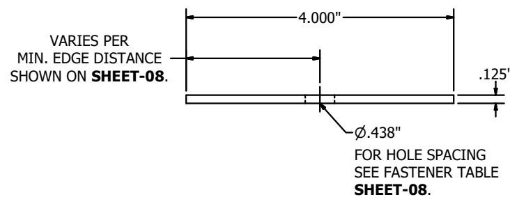
STIFFENER PLATE ITEM-24 N.T.S.
