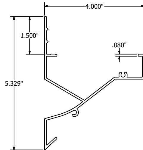
FLANGED HEAD FRAME ITEM-12 N.T.S.
