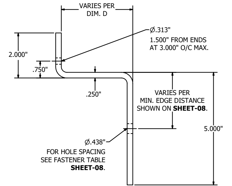
RETAINING ZEE ITEM-20 N.T.S.
