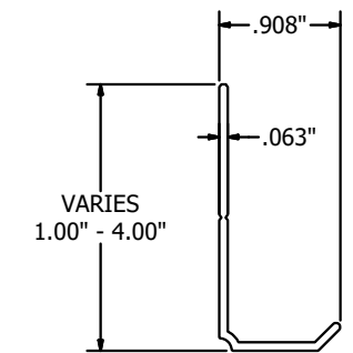
WATERSTOP ITEM-11 N.T.S.
