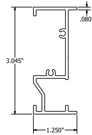
JAMB FRAME ITEM-3 N.T.S.
