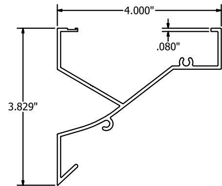
HEAD FRAME ITEM-7 N.T.S.
