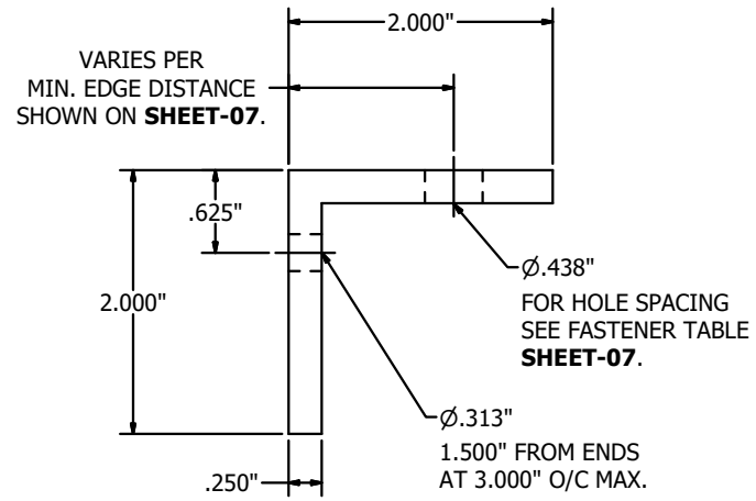
RETAINING ANGLE ITEM-15 N.T.S.
