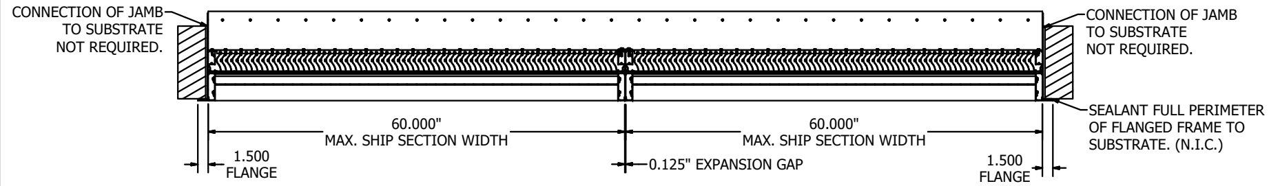
SECTION D-D
