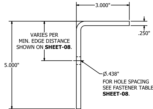
RETAINING ANGLE ITEM-22 N.T.S.
