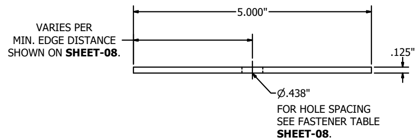
STIFFENER PLATE ITEM-23 N.T.S.
