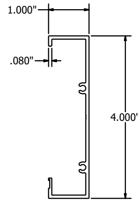
JAMB FRAME ITEM-9 N.T.S.
