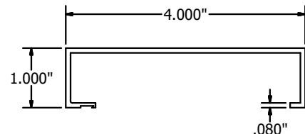
SILL FRAME ITEM-8 N.T.S.
