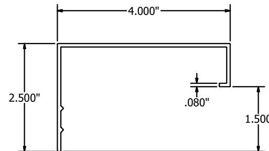
FLANGED SILL FRAME ITEM-13 N.T.S.
