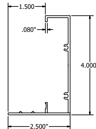
FLANGED JAMB FRAME ITEM-14 N.T.S.
